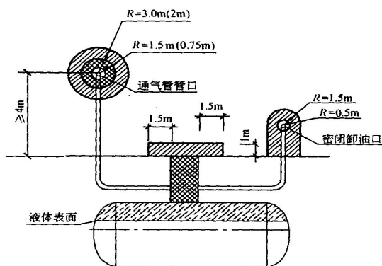
图 3.3-3 埋地卧式汽油储罐爆炸危险区域划分
