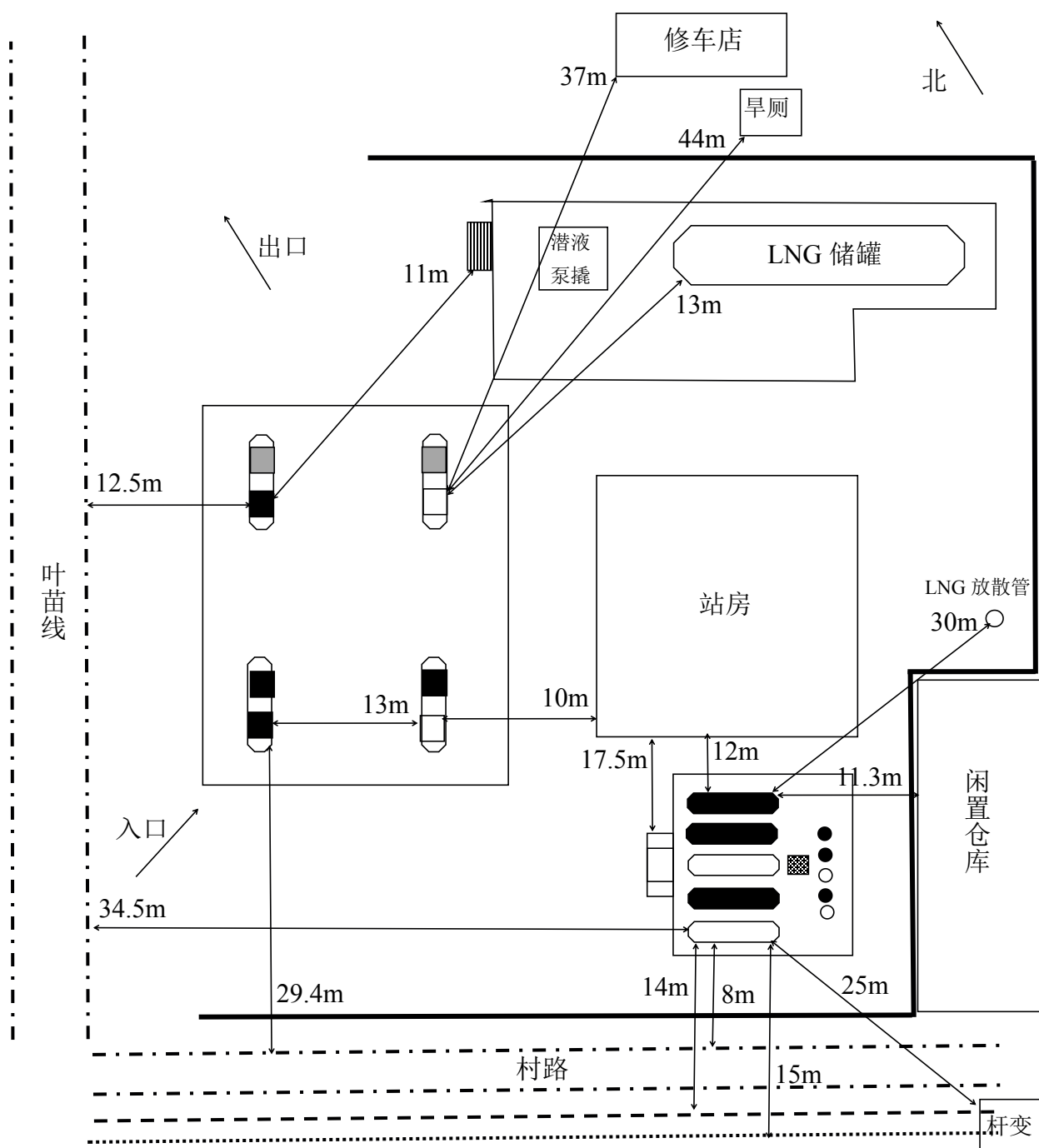
图 2.3-1 周边环境及总平面布置图
